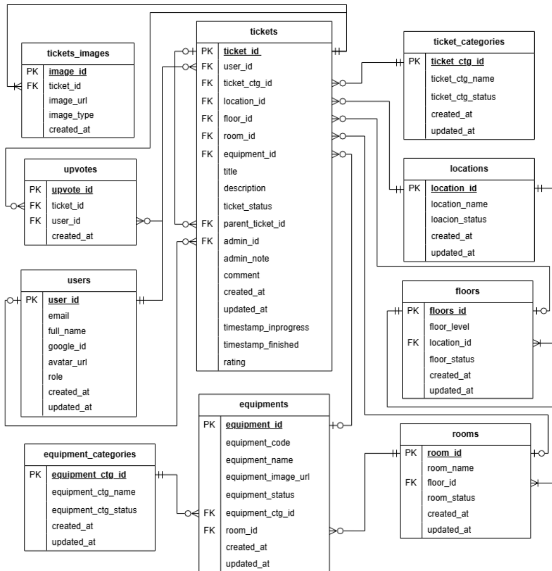
ภาพที่ 0.6 แผนภาพจำลองโครงสร้างข้อมูลของระบบติดตามปัญหา กรณีศึกษาวิทยาการคอมพิวเตอร์
