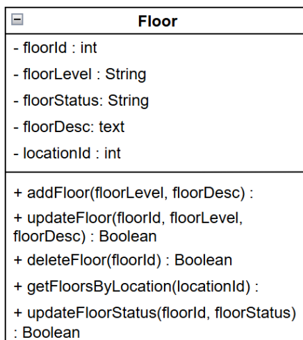
ภาพที่ 0.4 แผนภาพคลาสชั้น
